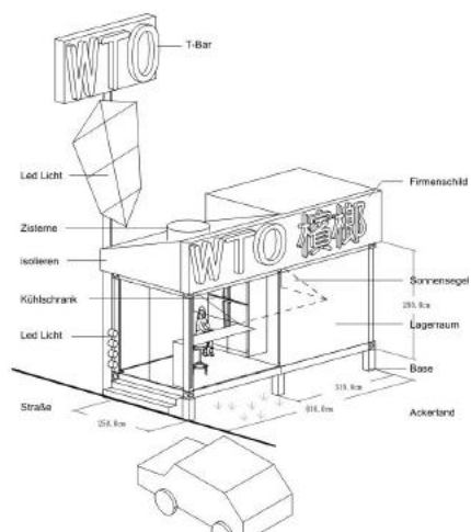
Elemente: T-Bar, Sonnensegel, LED-Licht, Zisterne, Lagerraum 構件：T 型桿、遮陽棚、LED 燈、水塔、儲藏室
