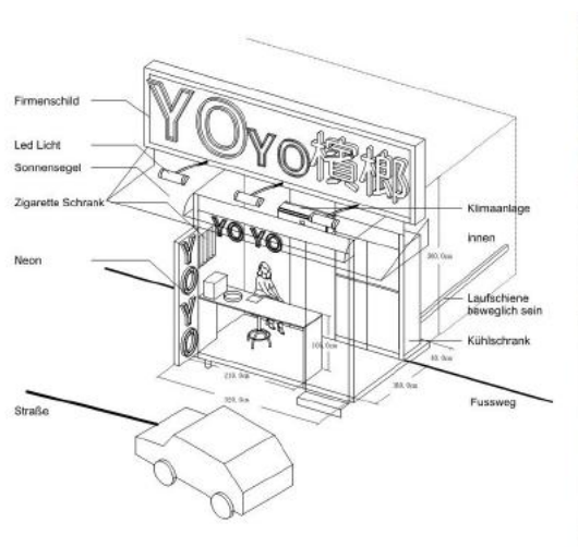
Elemente: Laufschiene, Neon, LED-Licht, Klimaanlage, Zigaretzenschrank 構件：滑軌、霓虹、LED 燈、冷氣、香菸櫃
