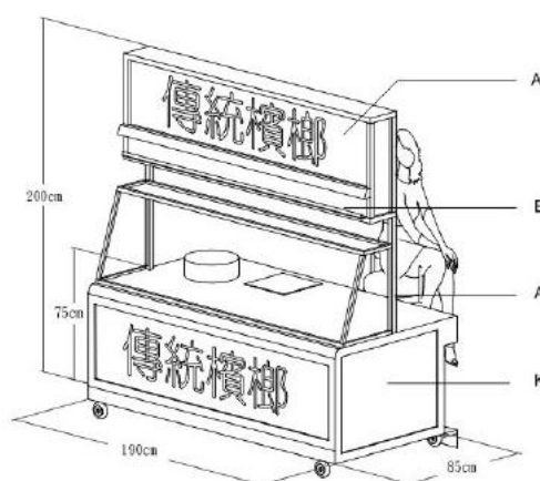
Elemente: Kühlschrank, Firmenschild, Anschlagzetteln, Arbeitstisch 構件：冰箱、招牌、價目表、工作檯
