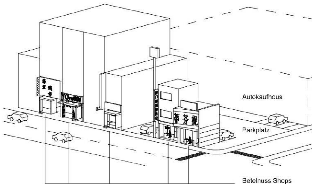
Axonometrie — Lage im Stadtraum 軸測圖——城市空間中的位置關係
